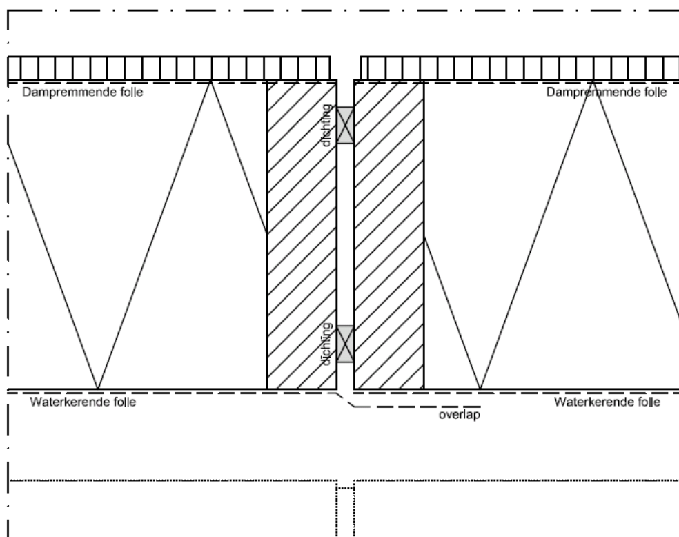
Detail binnenspouwblad
