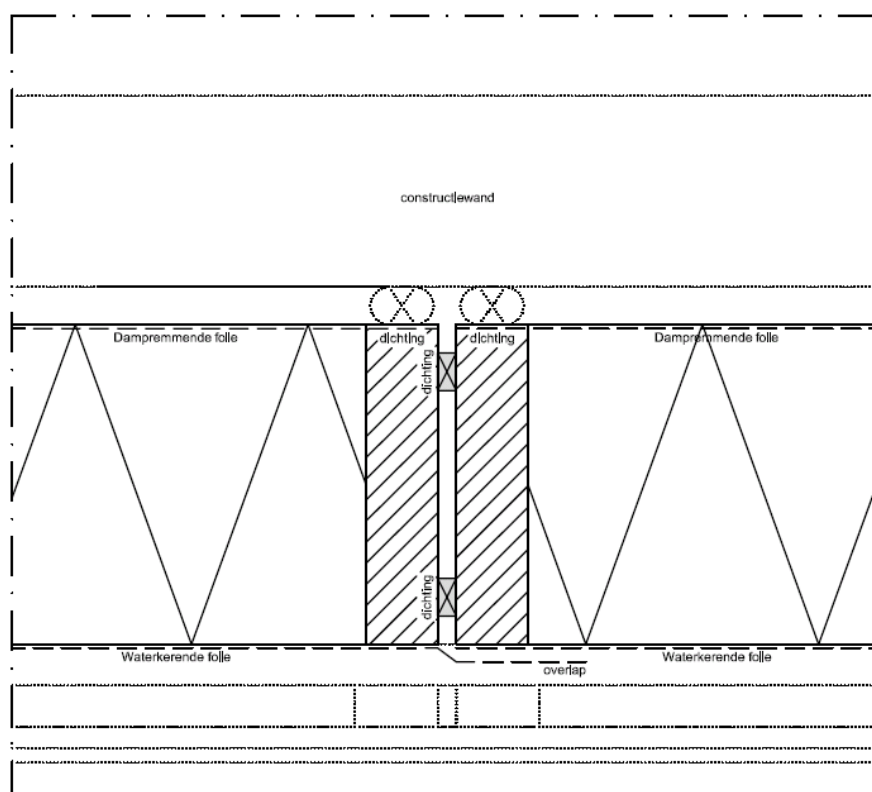
Detail voorzetwand
