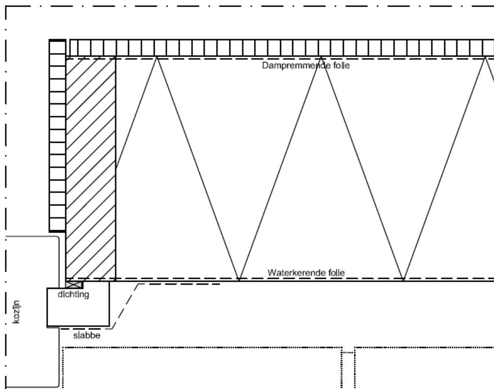
Detail binnenspouwblad
