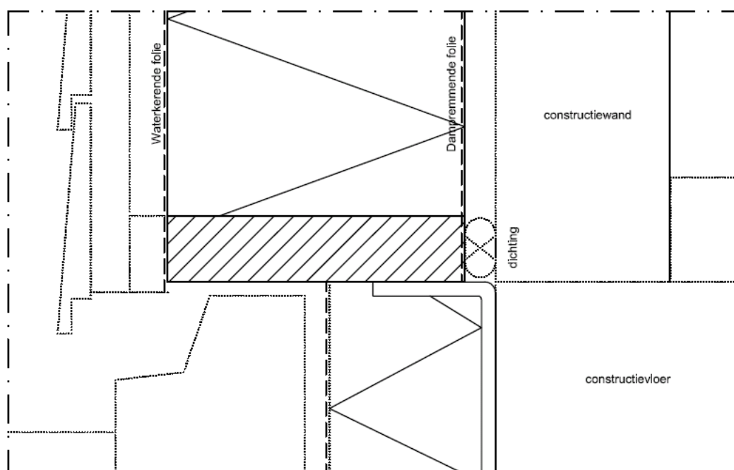
Detail voorzetwand
