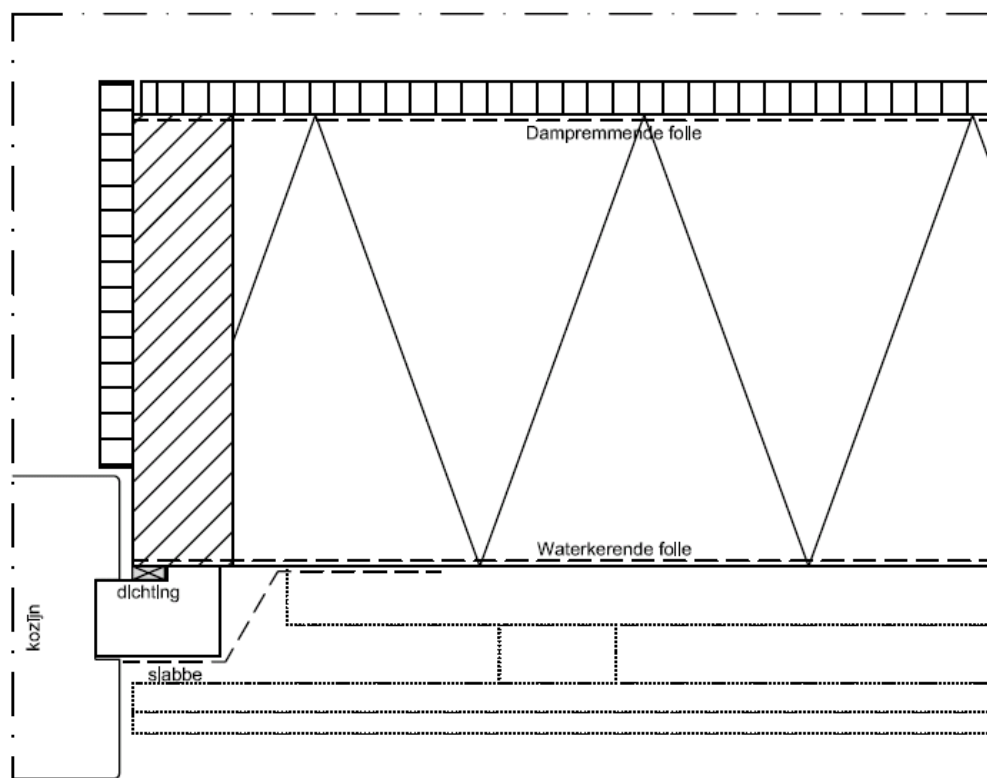
Detail gevelsluitend element
