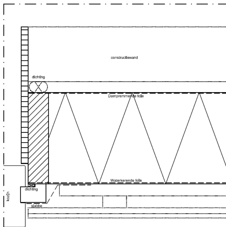
Detail voorzetwand
