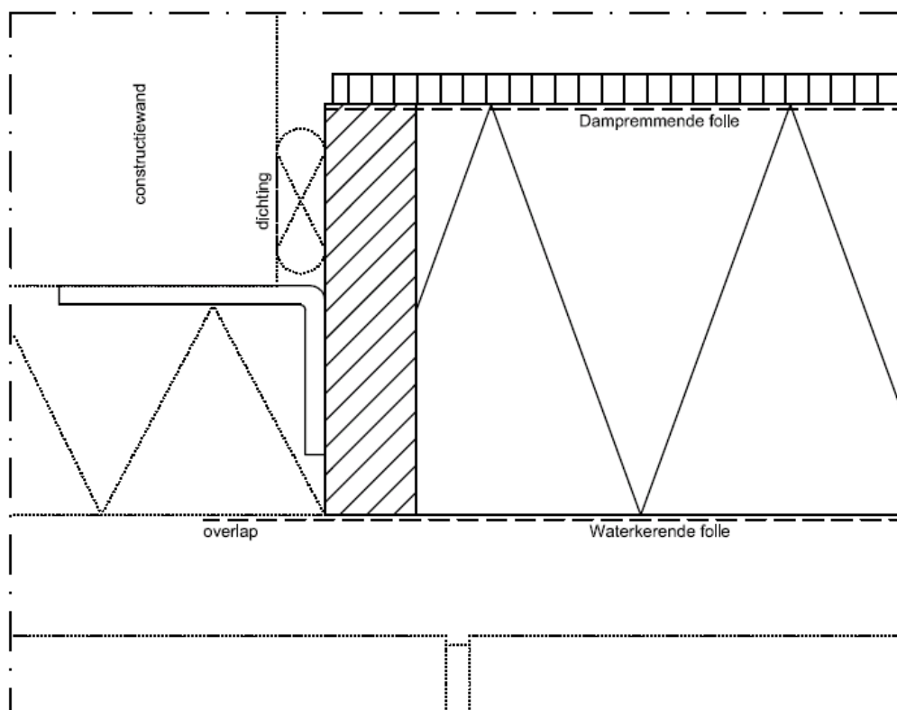
Detail binnenspouwblad
