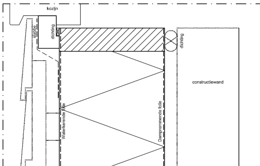
Detail voorzetwand
