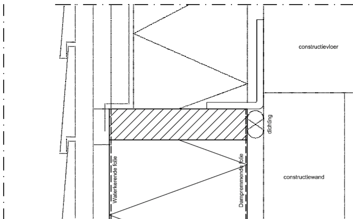
Detail voorzetwand
