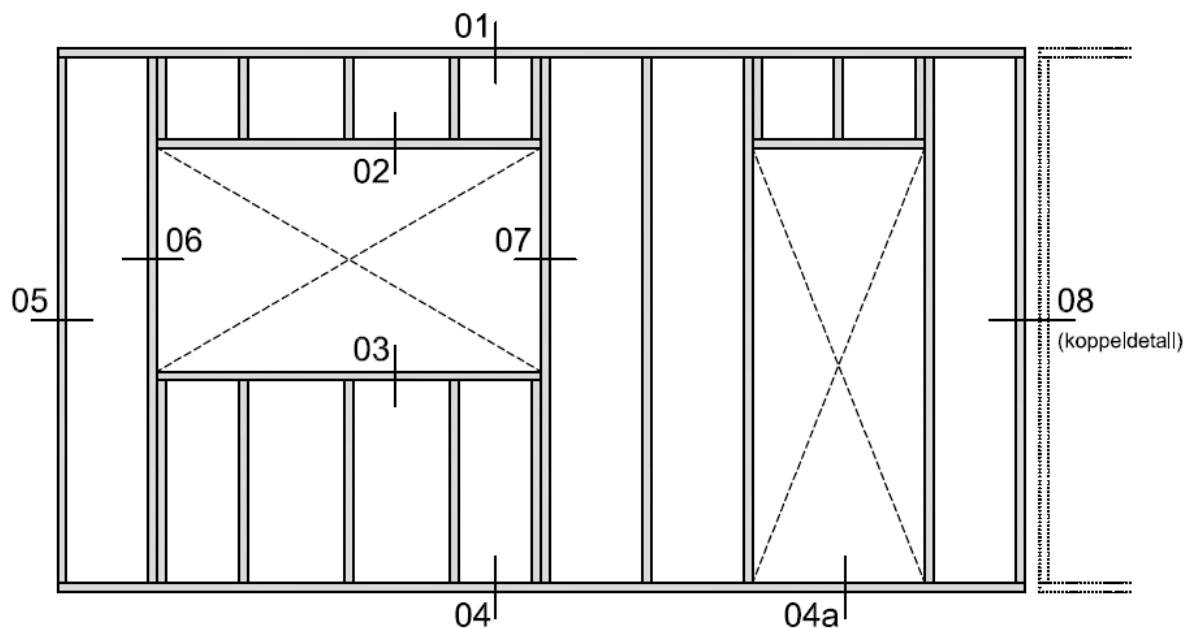
Bijlage 1 details binnenspouwbladen
