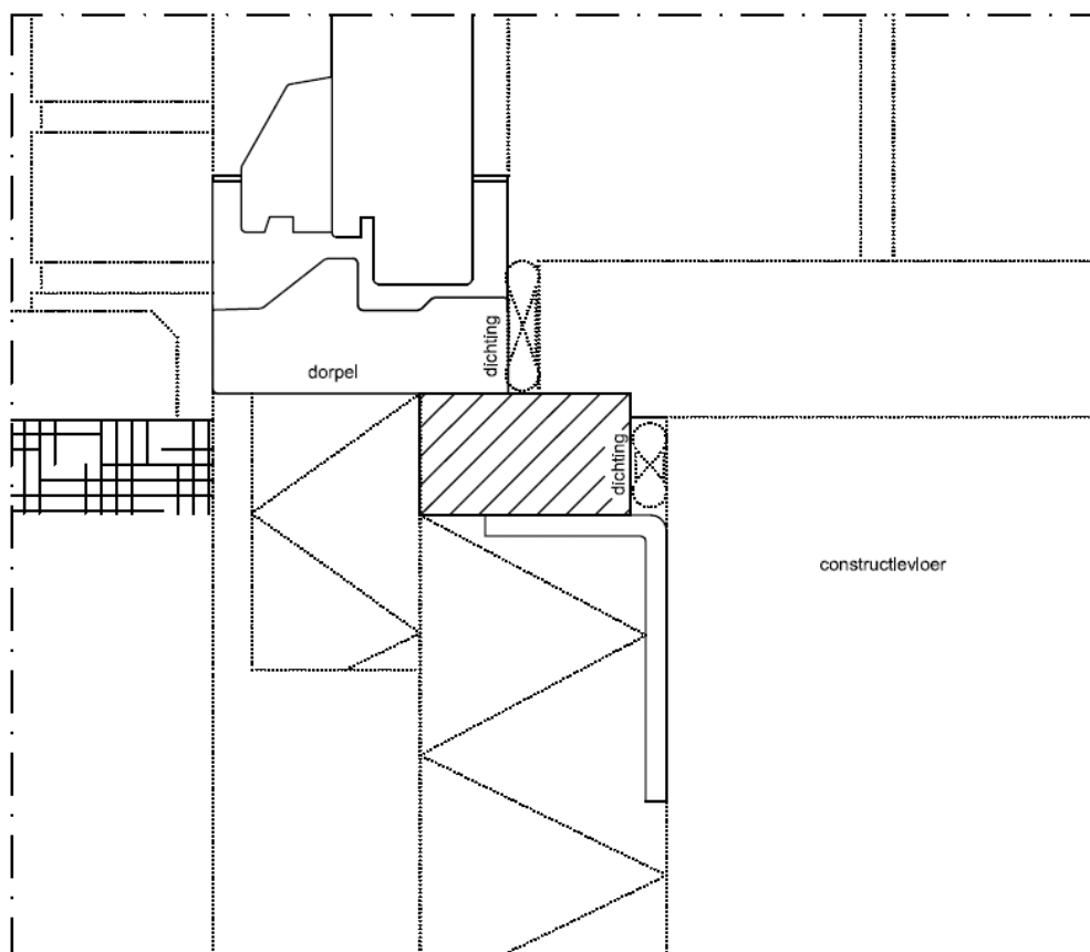
Detail binnenspouwblad
