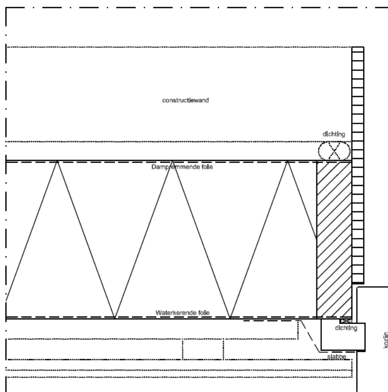
Detail voorzetwand
