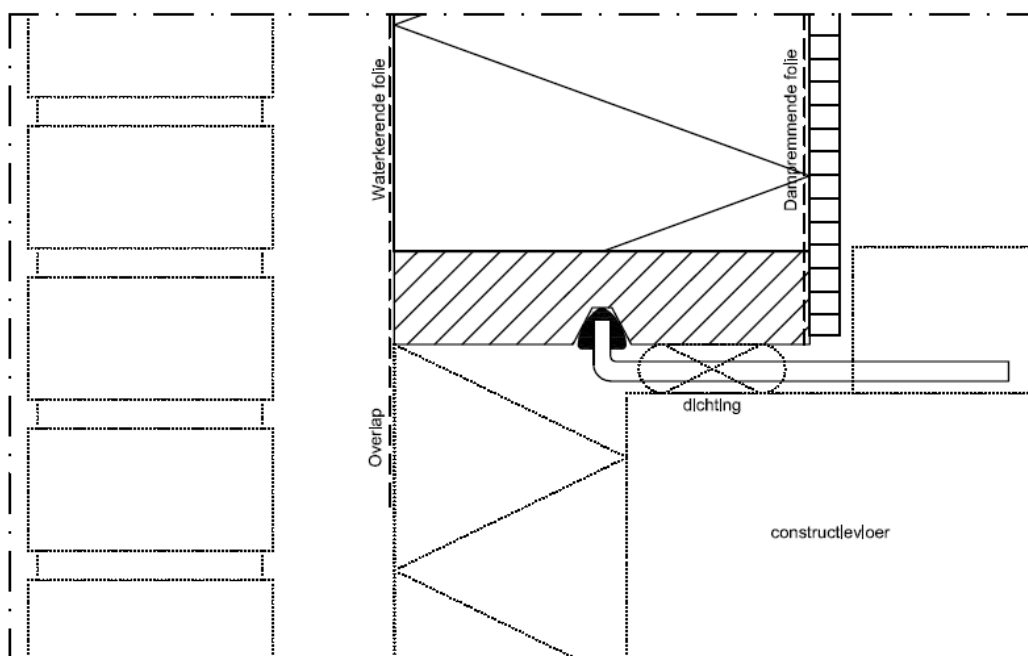
Detail binnenspouwblad
