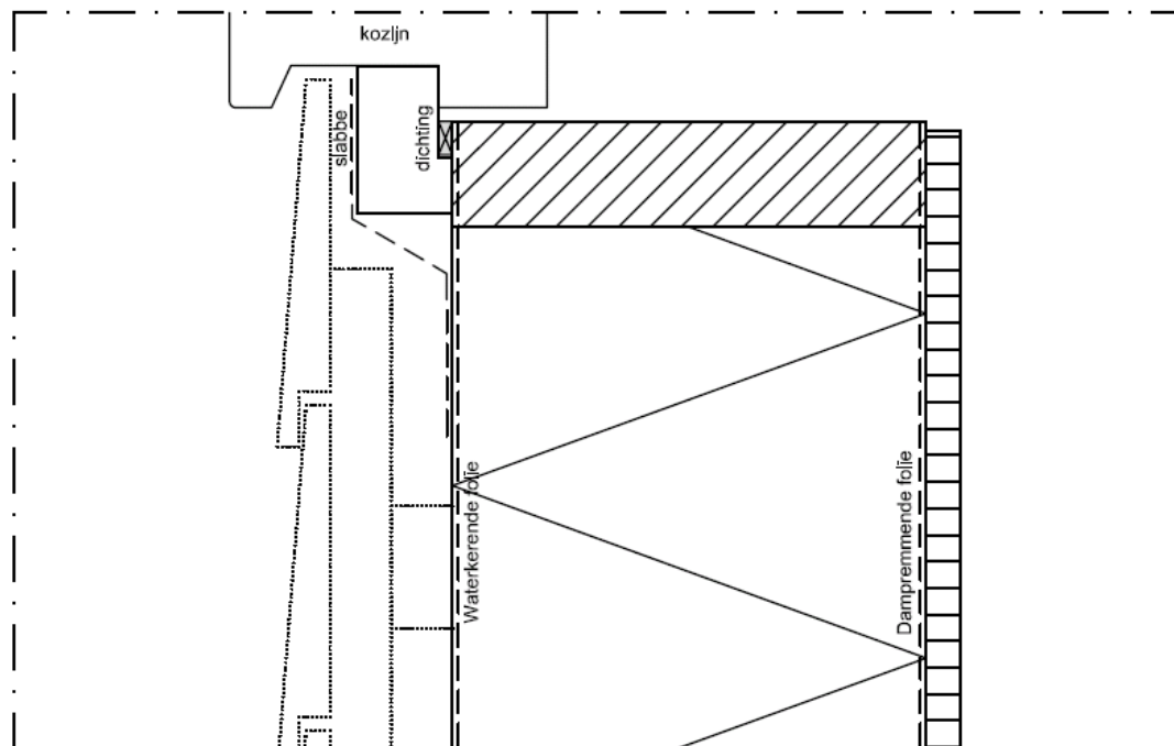
Detail gevelsluitend element
