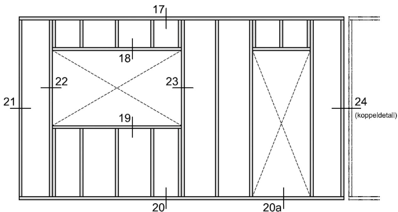
Bijlage 3 details voorzetwanden
