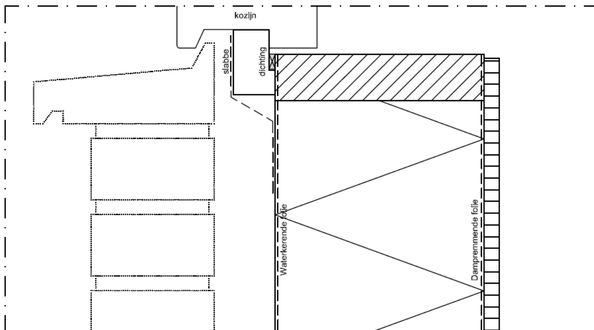
Detail binnenspouwblad
