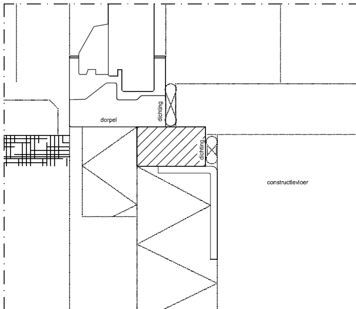
Detail voorzetwand
