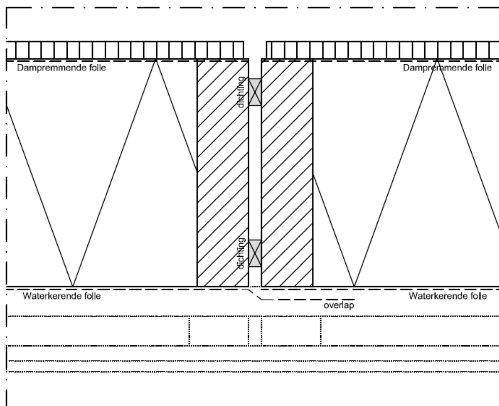
Detail gevelsluitend element
