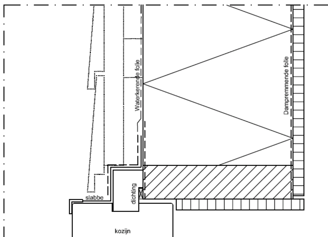
Detail gevelsluitend element
