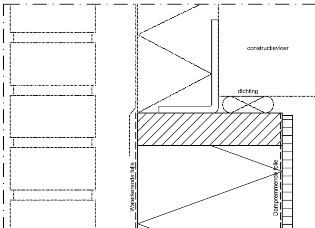
Detail binnenspouwblad
