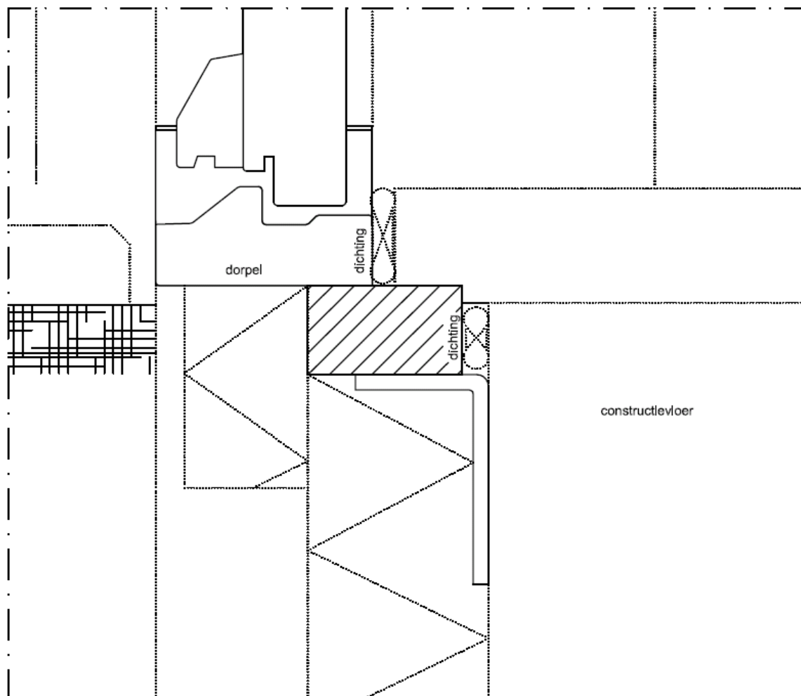
Detail gevelsluitend element
